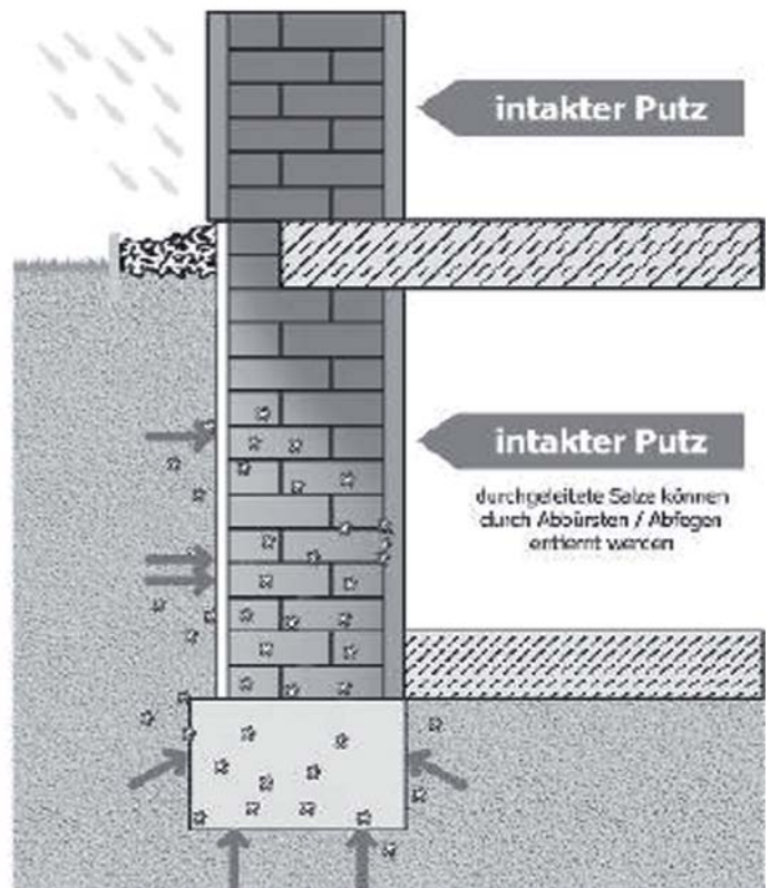
Feuchteregulierungsputz transportiert die Salze an die Oberfläche und der Putz platzt nicht ab.
