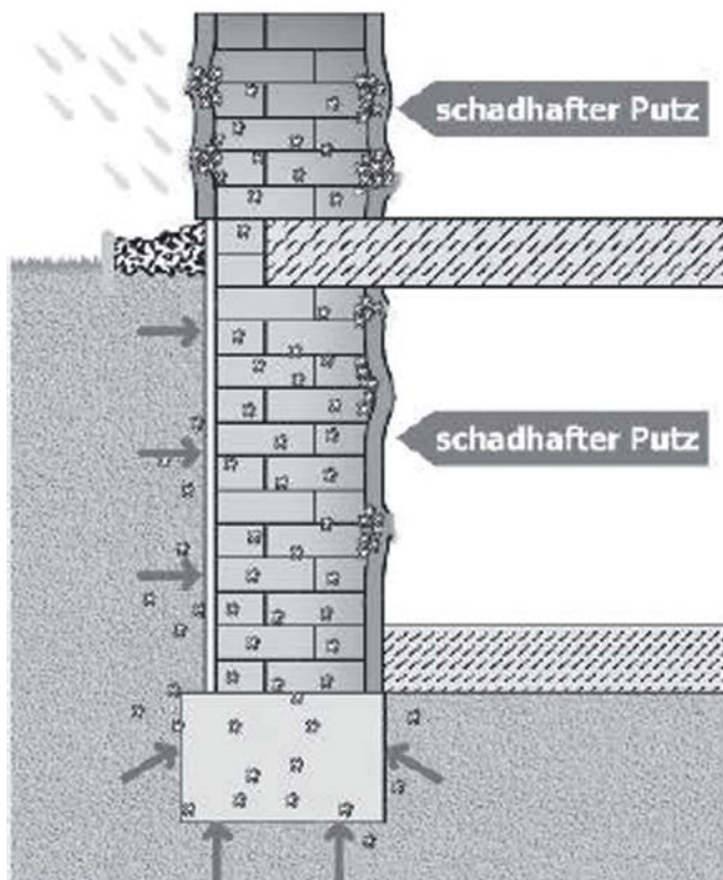
Sanierputz lagert die Salze ein und der Putz platzt ab.
